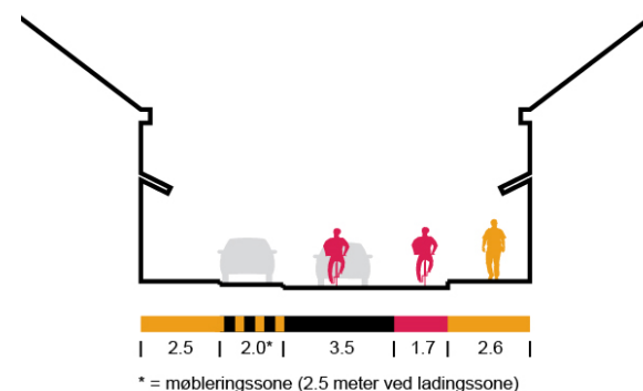
Foreslått snitt for Storgata (nord fra gågata)
