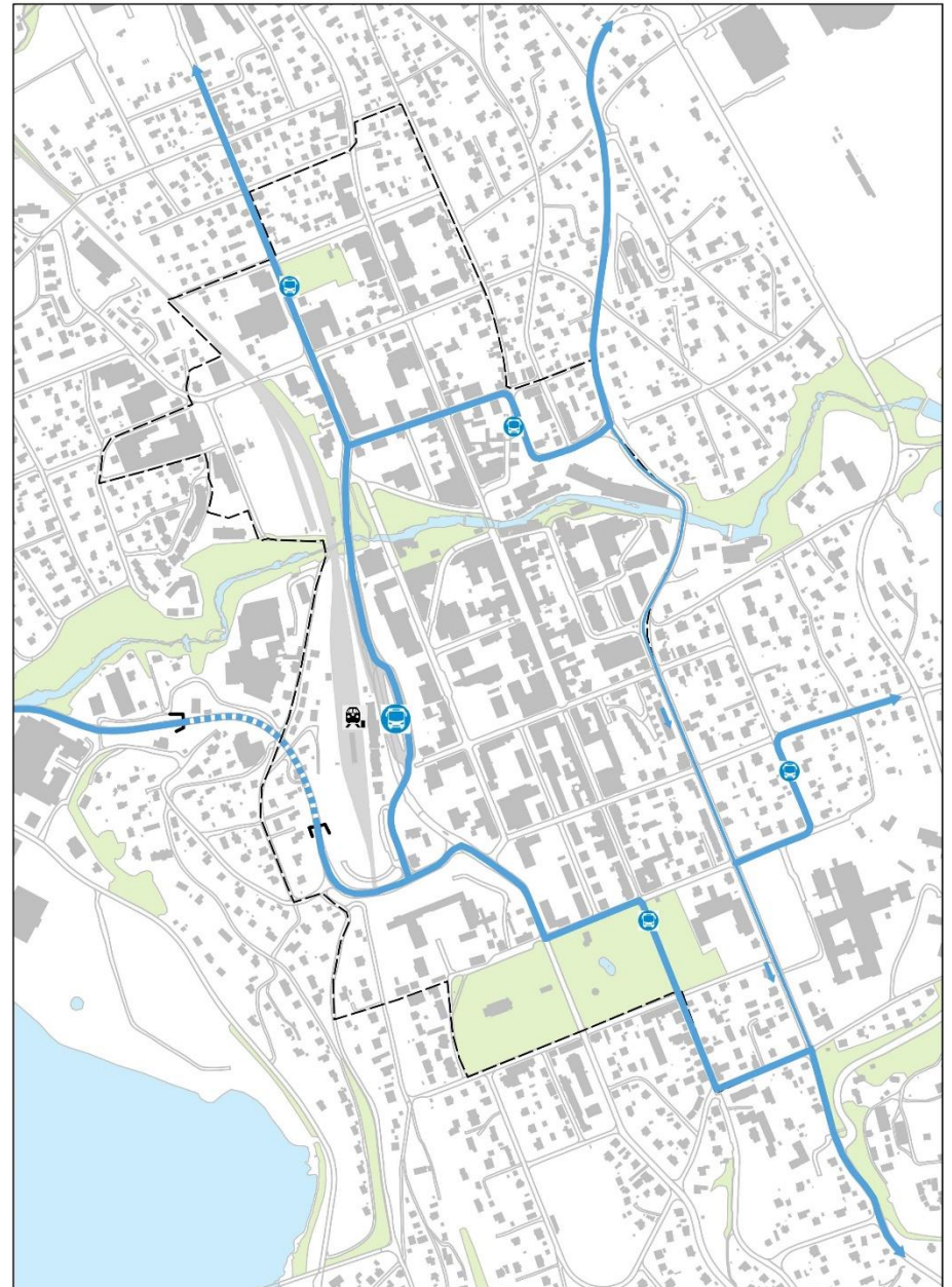
Figur 21 Trasé og holdeplass struktur med bussholdeplass i 2 retninger ved den gamle Brannstasjonen
