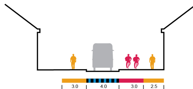
Alternativ for Anders Sandvig gate: Enveiskjøring for bil gir økt prioritering for gang og sykkel
