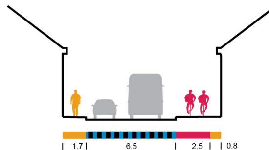
Foreslått snitt for Storgata (sør fra Søndre Park)
